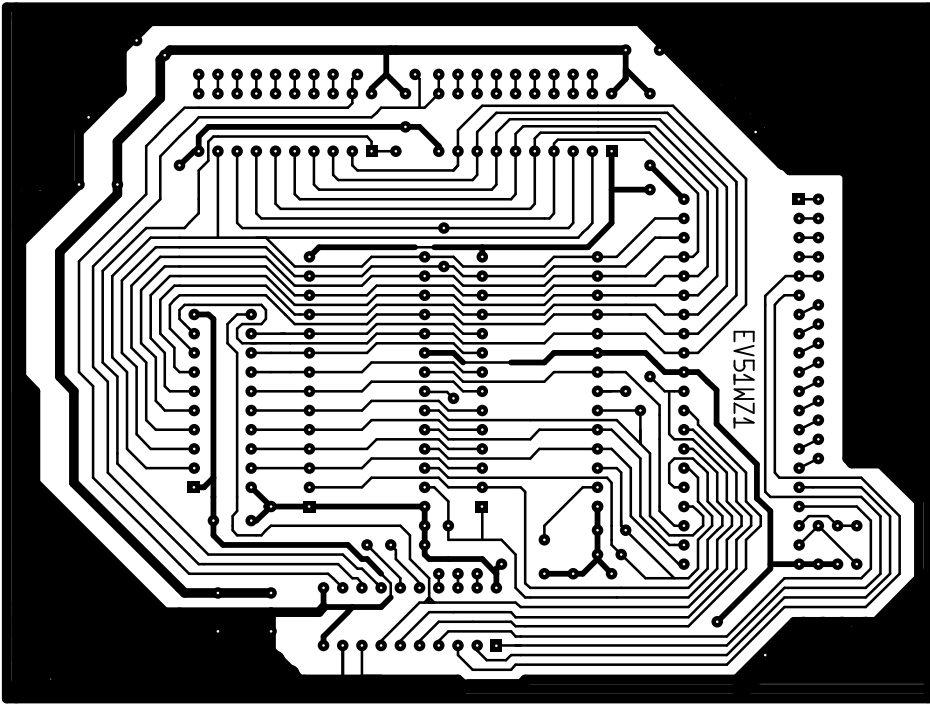
EV21M21 Bottom Layer
