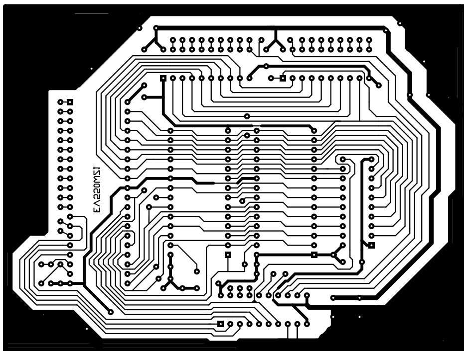
EV550WZ1 Bottom Layer
