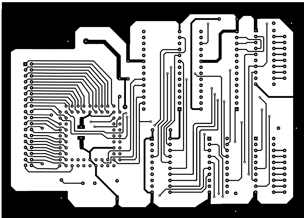
EV552WZ1 Bottom Layer
