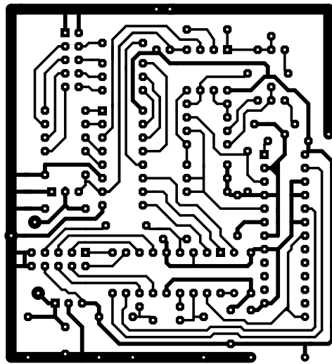
PICADC Bottom Layer
